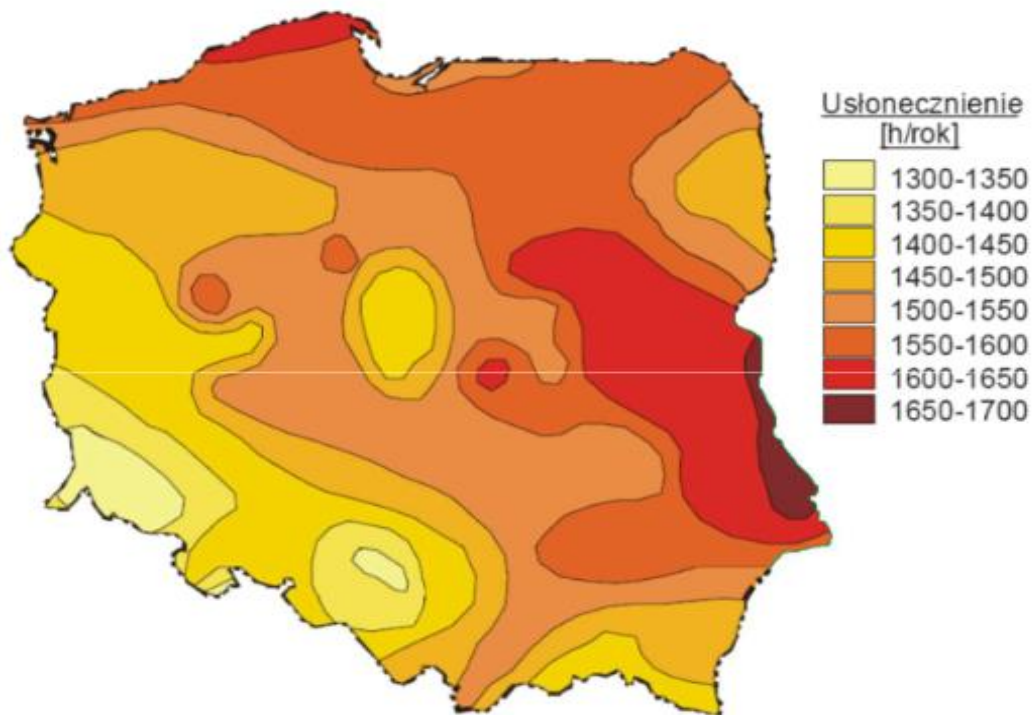
Rycina 6. Średnie roczne sumy usłonecznienia w Polsce
