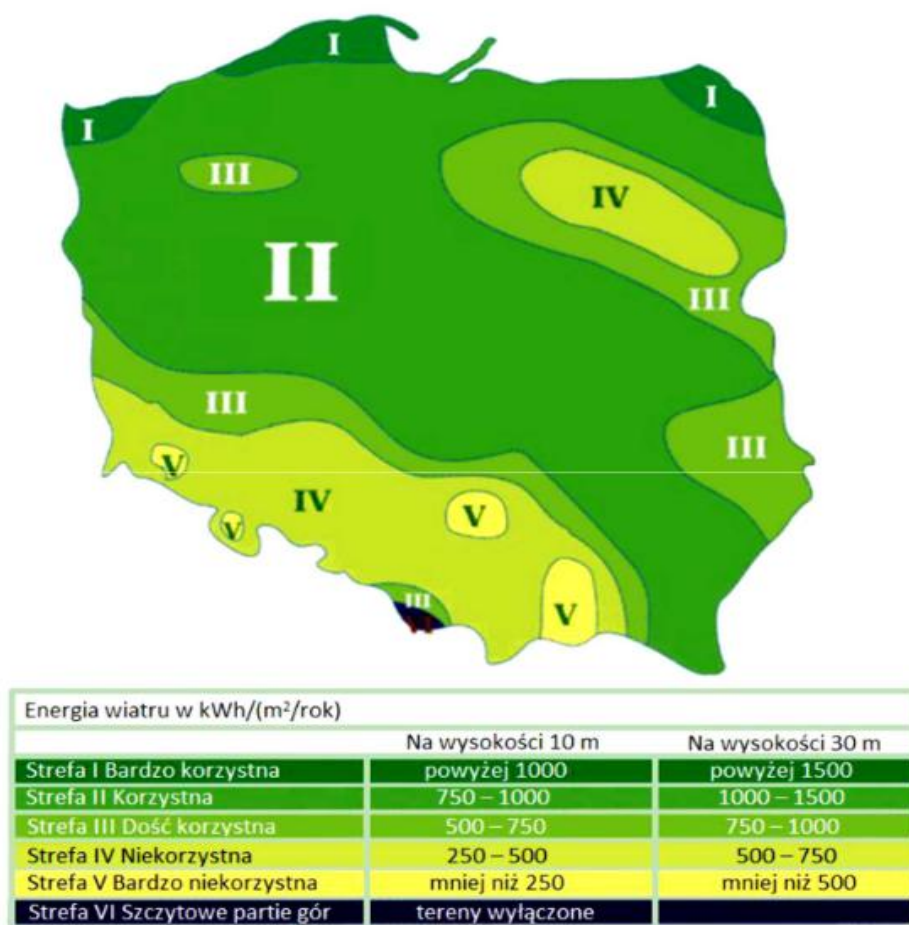
Rycina 5. Energia wiatru w Polsce w kWh/(m 2 /rok) na wysokości 10 i 30 metrów
