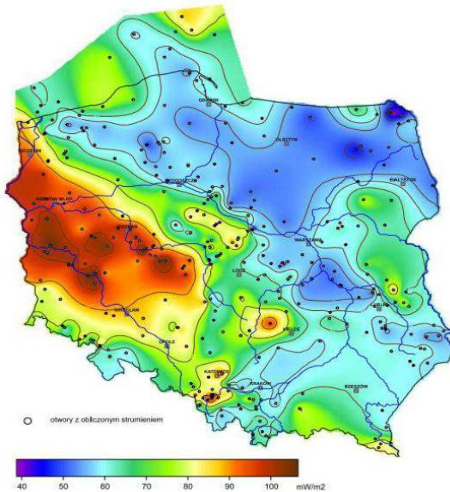
Rycina 7. Mapa rozkładu gęstości ziemskiego strumienia ciepłego na obszarze Polski
